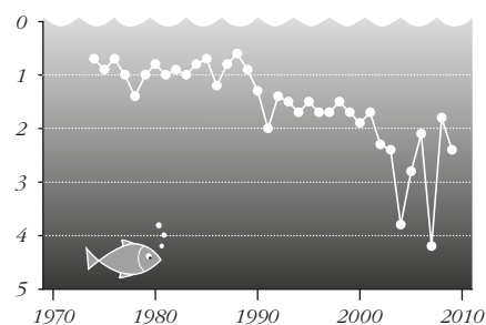
Siktdjup i meter i Brunnsviken. Sikten har förbättrats under den tid mätningar har gjorts. I dag kan sikten betecknas som måttlig.
